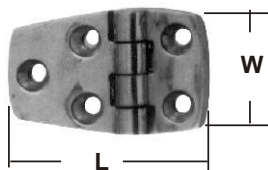
DOOR HINGE precision casted AISI 316
