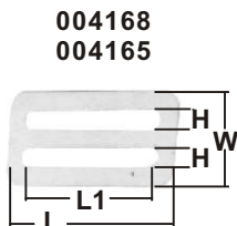
RECTANGULAR WEBBING SLIDES AISI 304
